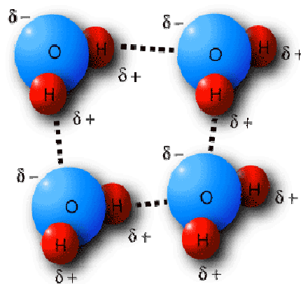
Fig. 4-4: Van der Waals Bonding
